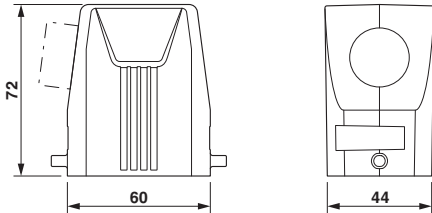
尺寸图
