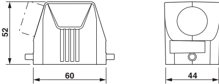
尺寸图
