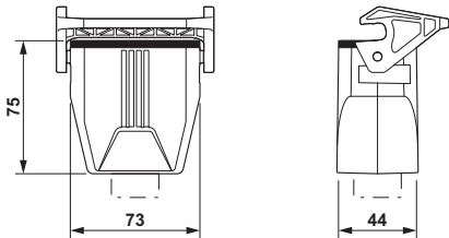
尺寸图
