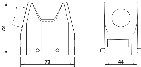
尺寸图
