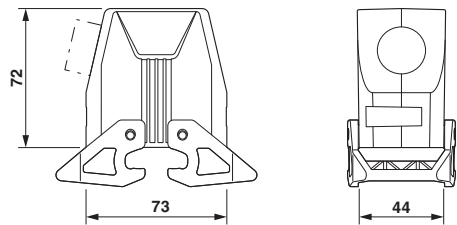
尺寸图
