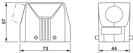
尺寸图
