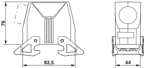
尺寸图
