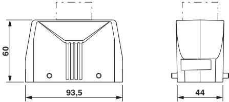
尺寸图
