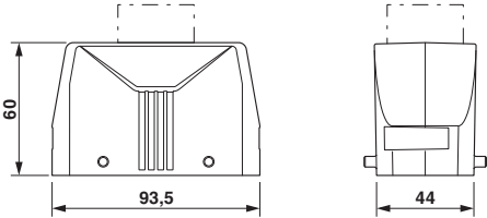
尺寸图
