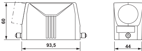
尺寸图
