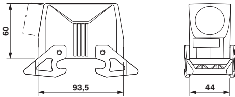
尺寸图
