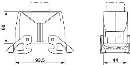
尺寸图
