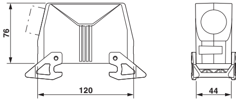
尺寸图
