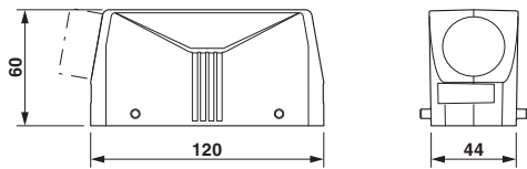
尺寸图
