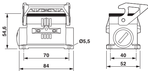
尺寸图
