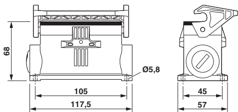
尺寸图
