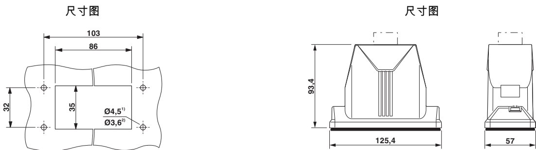
尺寸图
