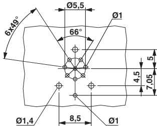
钻孔图
