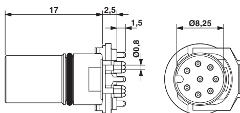
尺寸图
