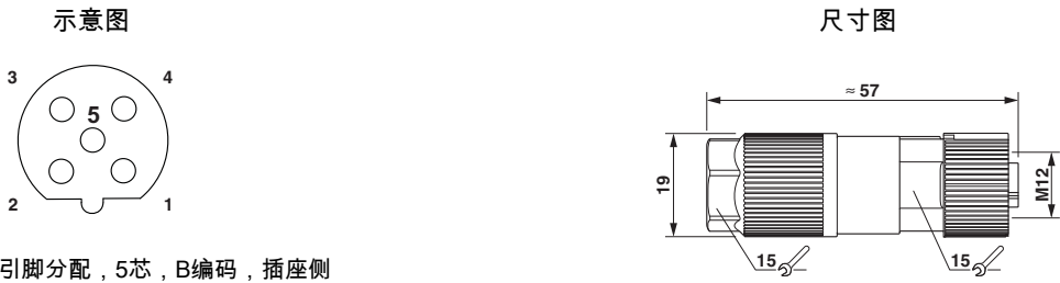
M12孔式连接器引脚分配，5芯，B编码，插座侧
