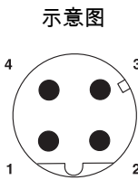
M12针式连接器引脚分配，4芯，D编码，插头侧
