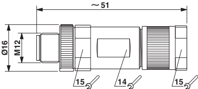
尺寸图
