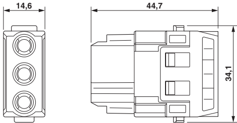
尺寸图
