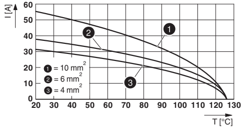
衰减曲线图 ( HC-B 24外壳可容纳6个模块 )
