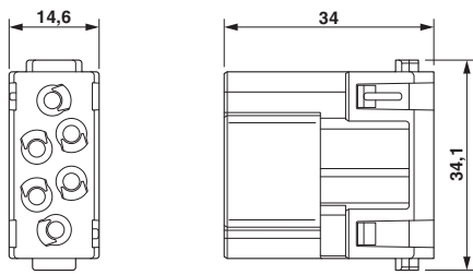
尺寸图
