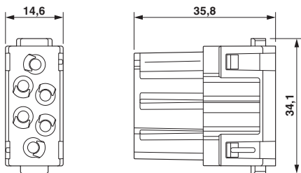
尺寸图
