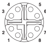
M12插座的引脚分配，8位，插座侧视图
