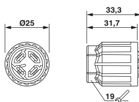
尺寸图
