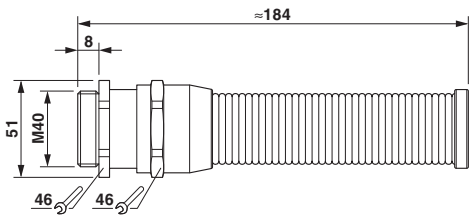
尺寸图
