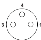
M8孔式引脚分配，3芯，插座侧视图
