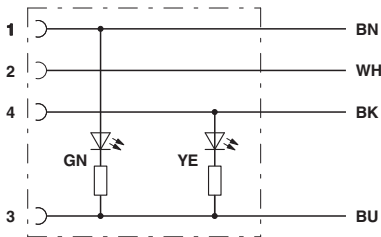
带LED的M8/M12孔式触点分配
