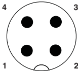
M12针式连接器引脚分配，4芯，A编码，插头侧视图
