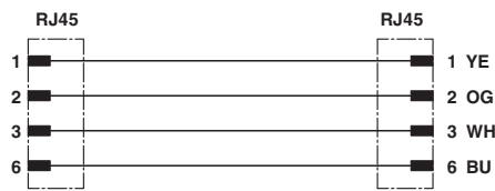
电路图
