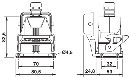
尺寸图
