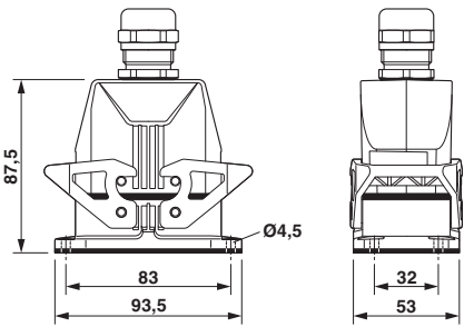
尺寸图
