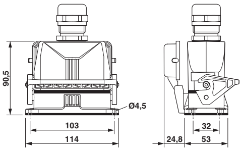
尺寸图
