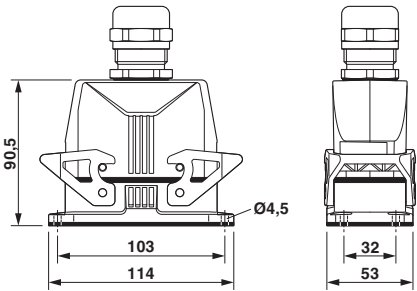
尺寸图
