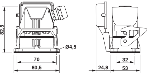
尺寸图
