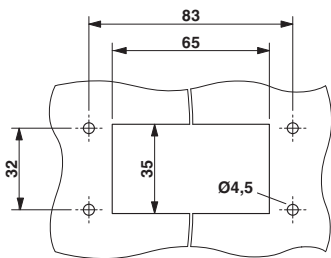
尺寸图
