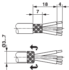
尺寸图
