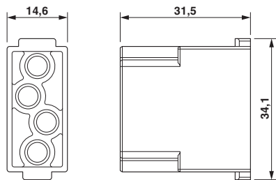
尺寸图
