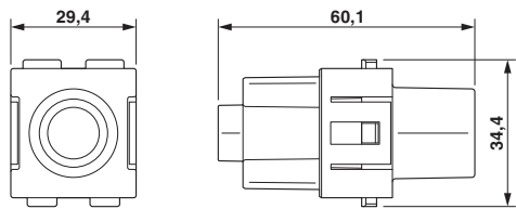
尺寸图
