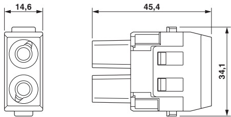
尺寸图
