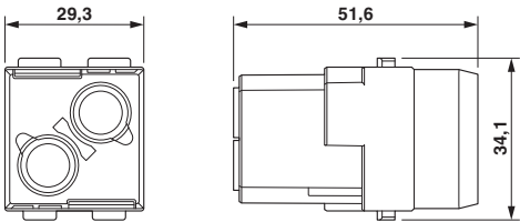
尺寸图
