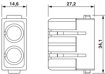
尺寸图
