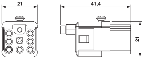
尺寸图
