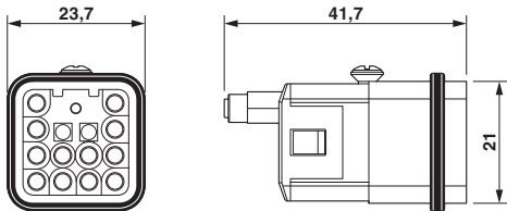
尺寸图
