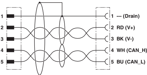
电路图
