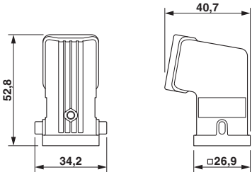
尺寸图
