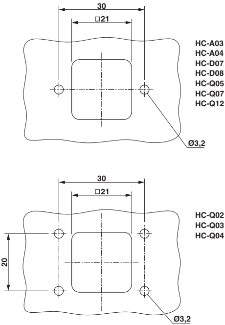
尺寸图
