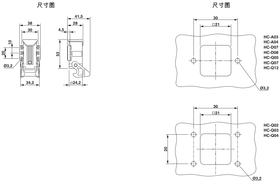
面板开口
