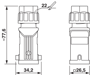
尺寸图
