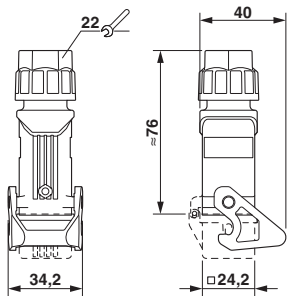
尺寸图
